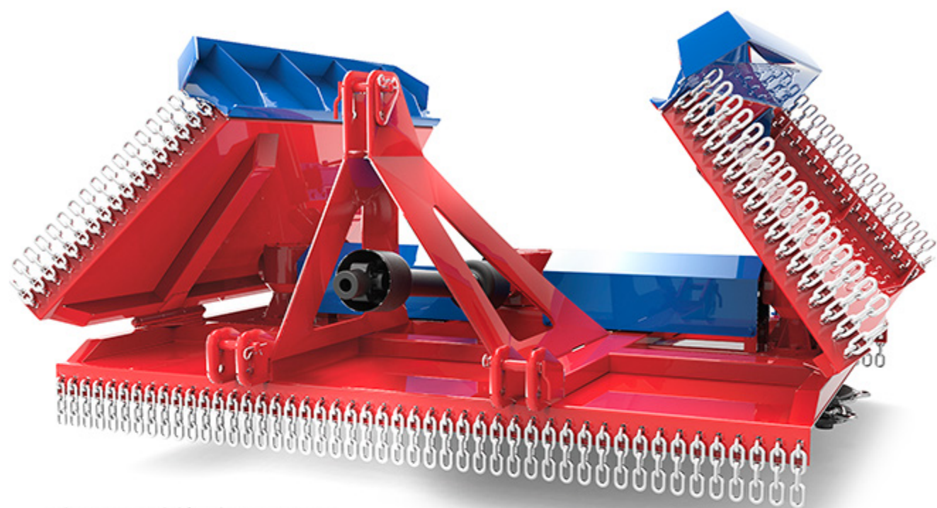
Vista en posición de transporte
